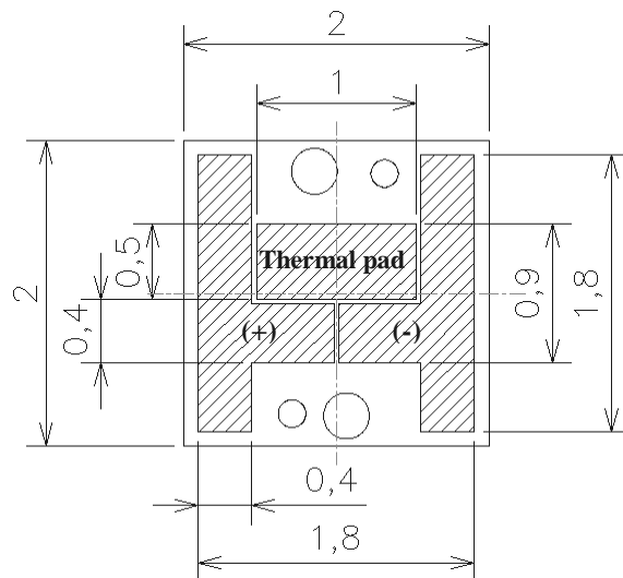
Cu pattern
