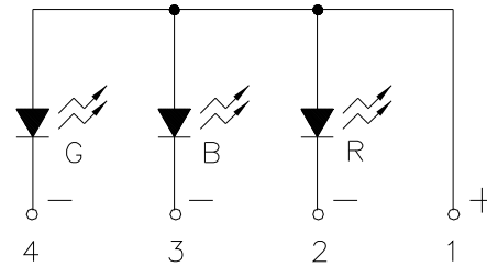
Polarity
